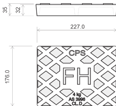
HYDRANT BOX LID
